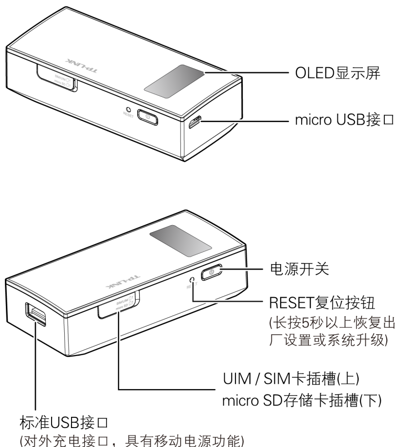
图 3.1 产品示意图
