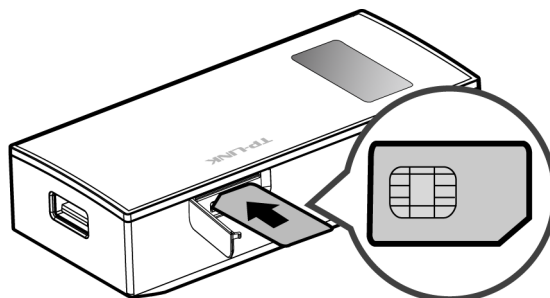
图 4.4 安装 UIM/SIM 卡
